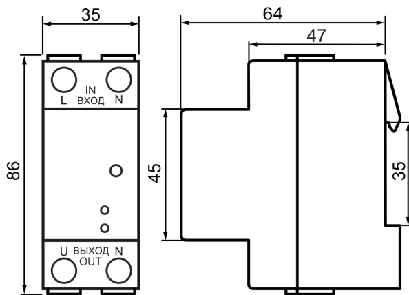
Габаритные размеры
